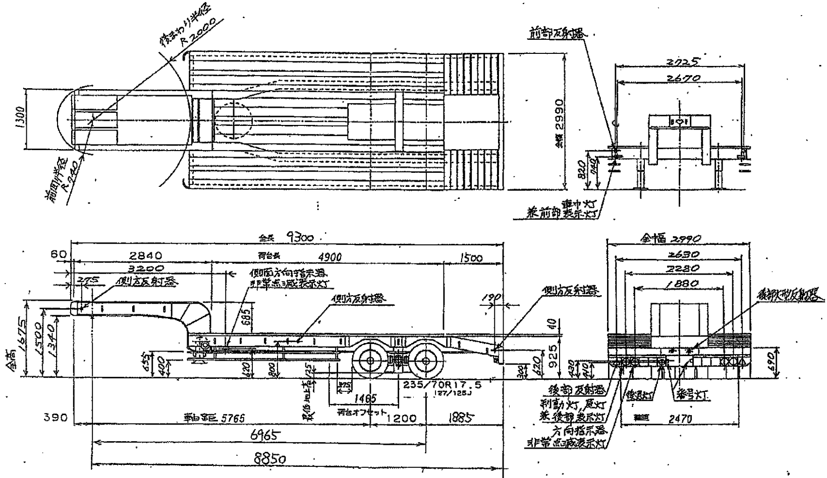
トールモービル PLR 431AH 型 外觀四面図
